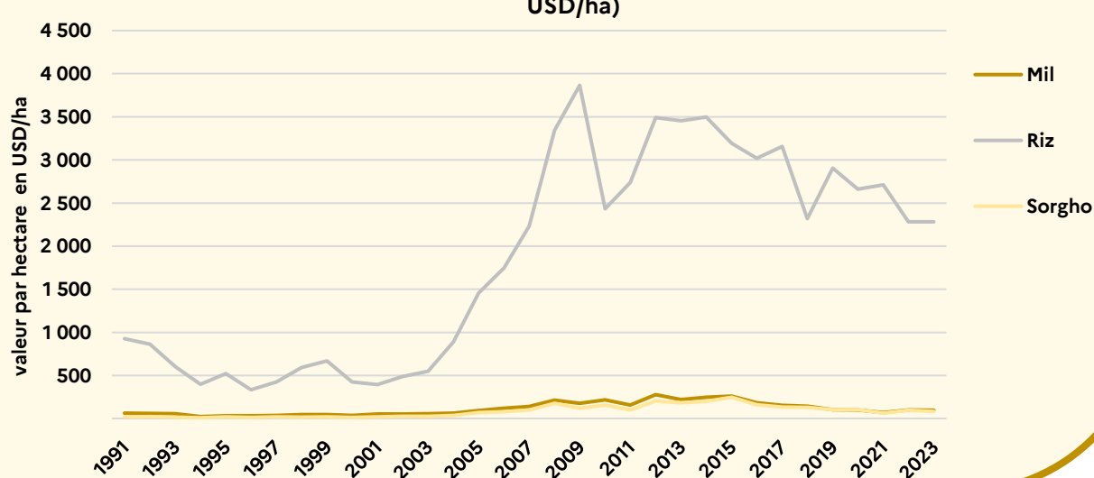
Évolution de la valeur de production de céréalière par hectare de plantation (en USD/ha)
