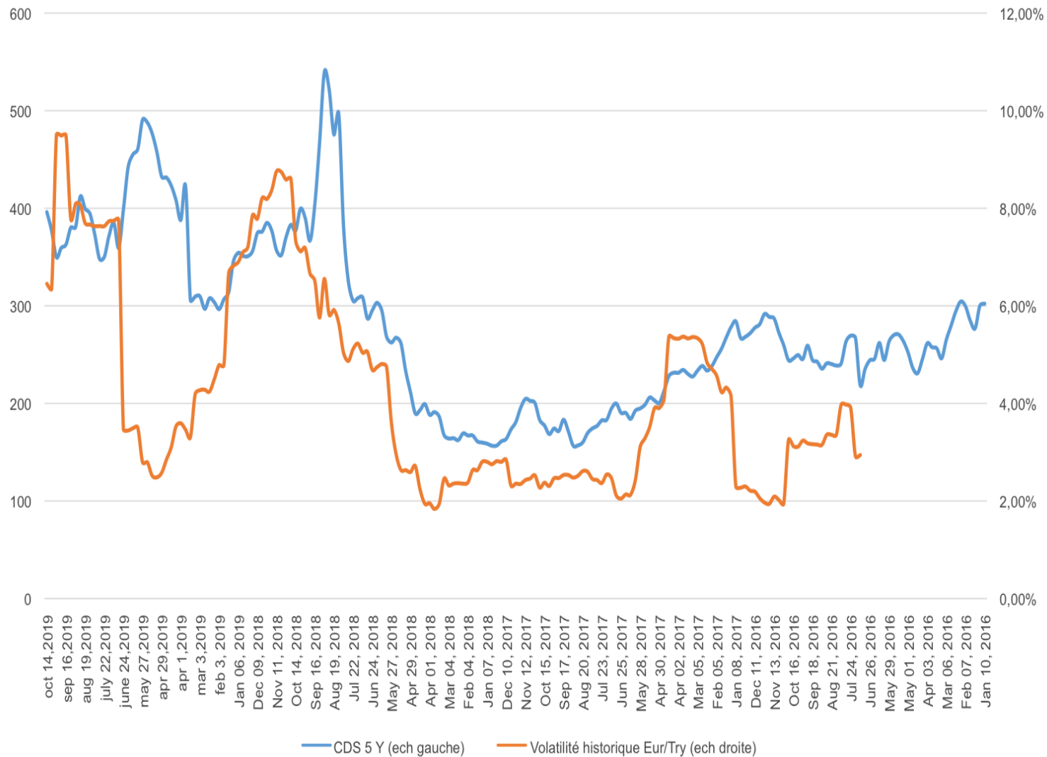
Evolution des indicateurs de risque (CDS et volatilité historique 3MM Eur/Try)
